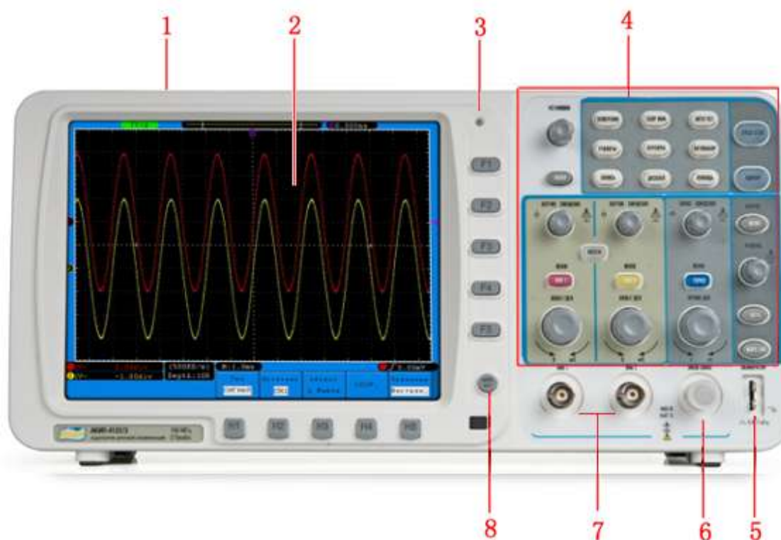
Рис. 6-1 Передняя панель осциллографов серии АКП-4122
