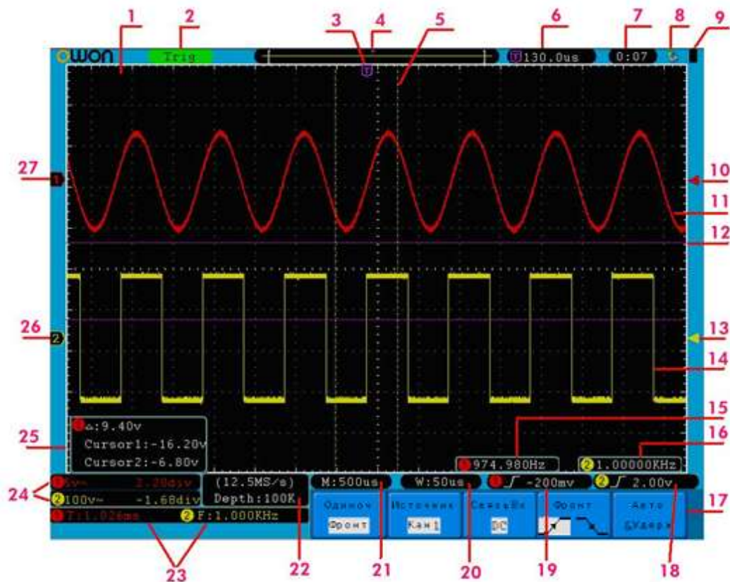
Рис. 6-6 Окно осциллографа АКІП-4122
