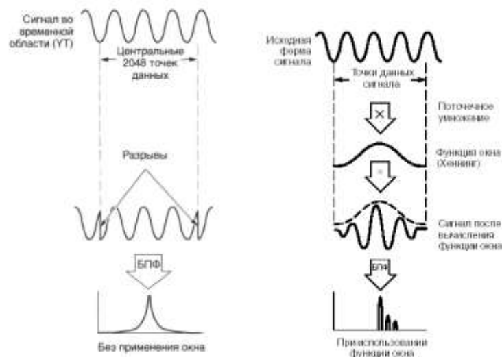
Рис. 8-6 Использовании функции окна в БПФ
